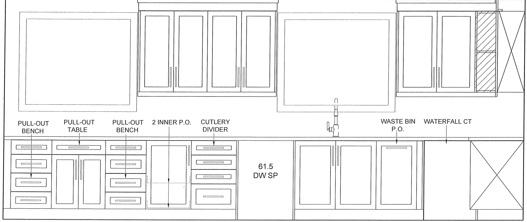
ELEVATION A
